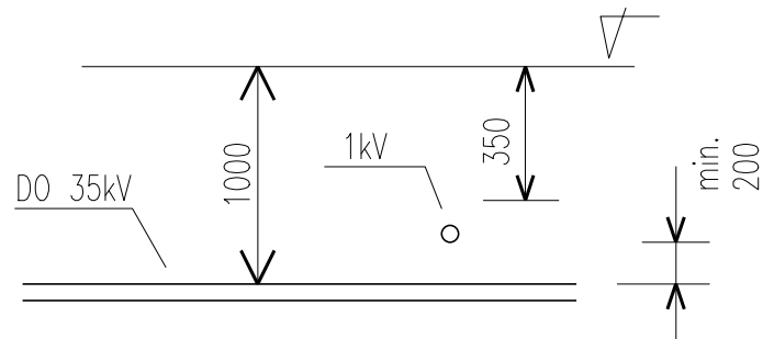
KŘÍŽENÍ KABEL 1kV/DO 35kV
