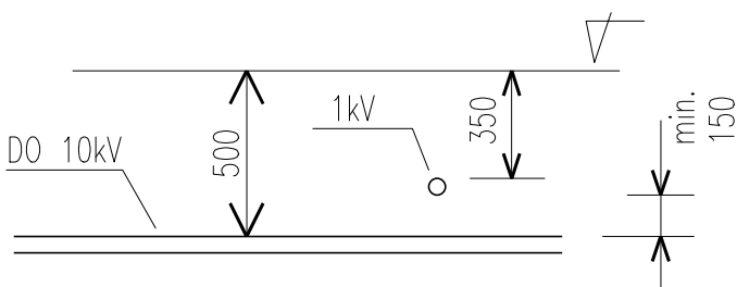
KŘÍŽENÍ KABEL 1kV/DO 10kV
