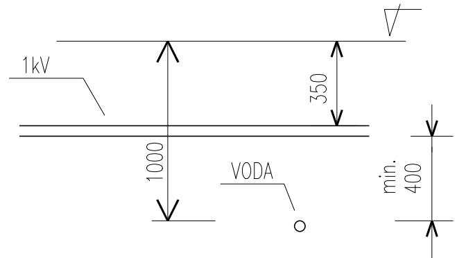
KŘÍŽNÍ KABEL 1kV/VODOVOD CHODNÍK – VOLNÝ TERÉN
