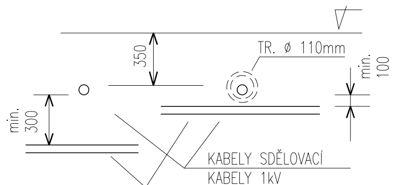
KŘÍŽENÍ SE SDĚLOVACÍMI KABELY
