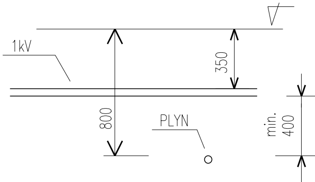
KŘÍŽENÍ KABEL 1kV/PLYN CHODNÍK – VOLNÝ TERÉN
