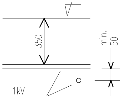
CHODNÍK KŘÍŽENÍ KABEL 1kV/1kV
